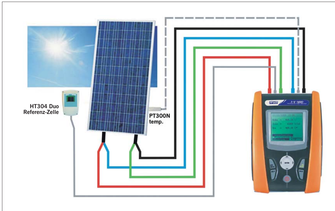
Anschlußdiagramm PV-Modulprüfung mit dem I-V400
