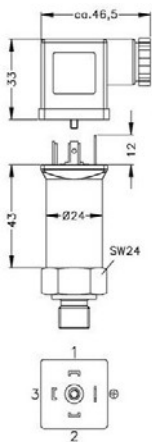
ISO 4400 (IP 65)
