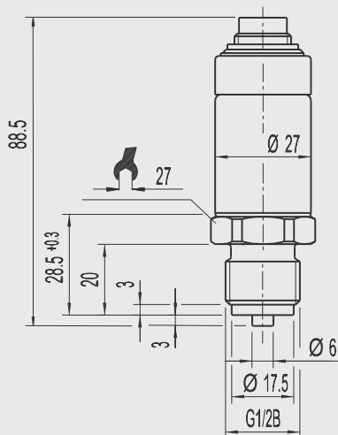
Referenz-Drucksensor CPT6200
