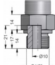
G1/2" DIN 3852 open port, P_N \leq 40 bar
