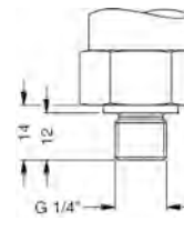
G1/4" DIN 3852
