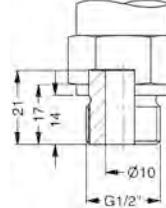
G1/2" offener Anschluss, P N ≤ 40
