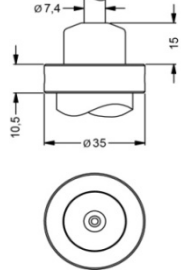
Kabelausgang, Kabel mit Belüftungsschlauch (IP68) 4
