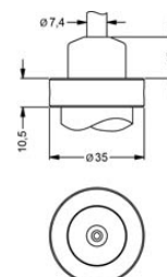
Kabelausgang, Kabel mit Belüftungsschlauch (IP 68) 6
