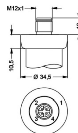
M12x1 4-polig (IP 67)
