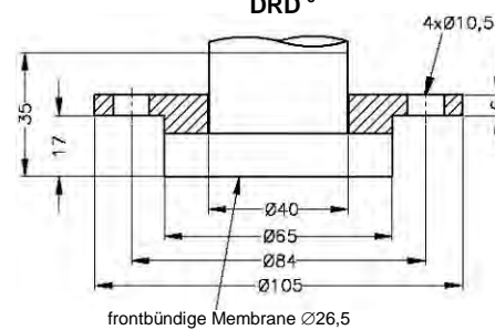
frontbündige Membrane Ø26,5
