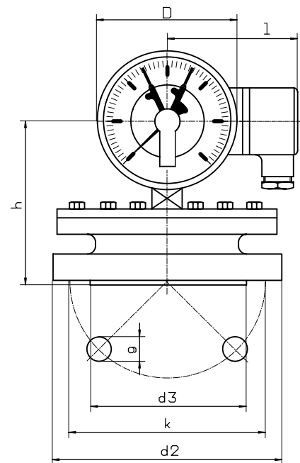
Messflansch 160 mm
