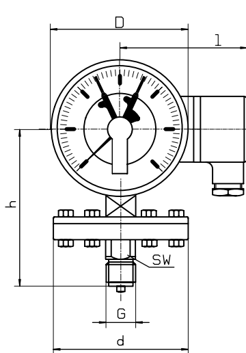
Messflansch 100 mm
