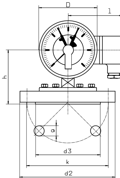
Messflansch 100 mm
