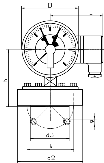
Messflansch 100 mm
