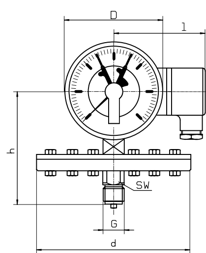
Messflansch 160 mm
