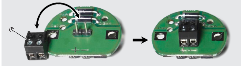
Abziehbare Schraubklemme
