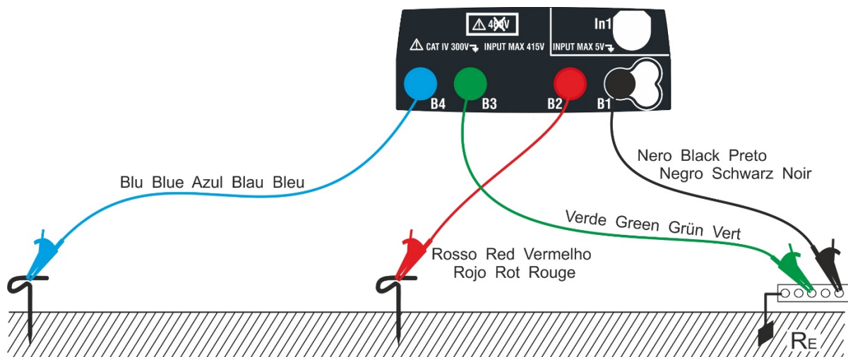
Abb. 28: 3-Punkt Erdungsmessung
