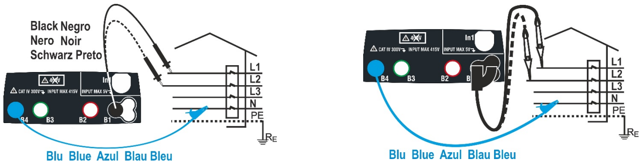
Abb. 25: Geräteanschluss zur Messung der Drehfeldrichtung mit zwei Messkabeln und Tastkopf
