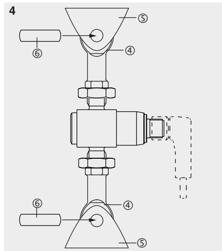
4 Gelenkköpfe in Haltevorrichtungen positionieren und mit Haltebolzen fixieren. Die Haltebolzen dürfen die freie Lagerung des Kraftaufnehmers nicht beeinträchtigen. Kraftaufnehmer belasten.
