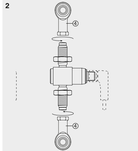
2 Gelenkköpfe auf Gewinde aufschrauben.
