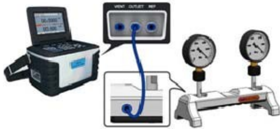
Kalibrierung von Manometer (mit Adapterblock)
