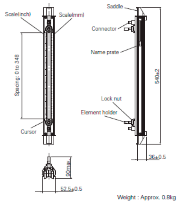
Detector FSSD3
