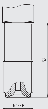
Hochdruck-Prozessanschluss (HP) für Anschluss mit Dichtlinie, nach EN 837
