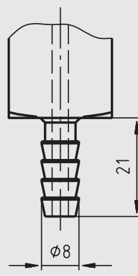
Schlauchanschluss
