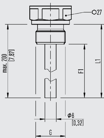
DIN EN ISO 1179-2 (ehemals DIN 3852-E)
