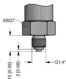
G1/4" EN 837
