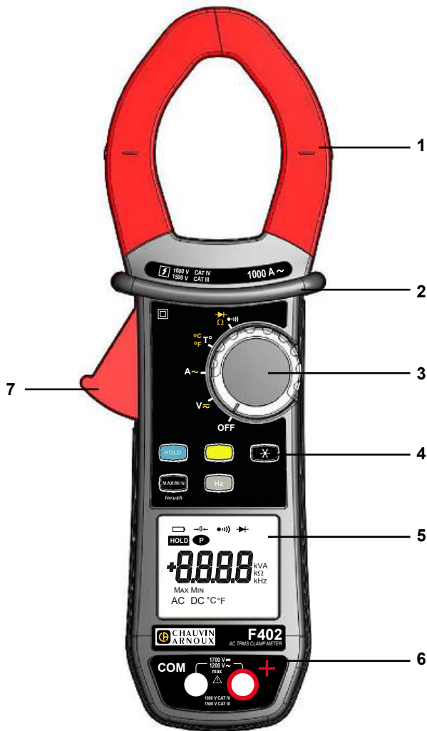
Abbildung 1: Vielfachmesszange F402
