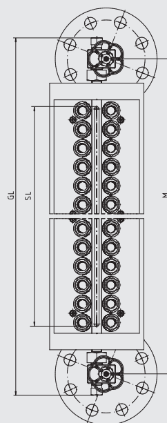
Ausführung mit Ventilkopf, oben/unten, Typ LGV-53
