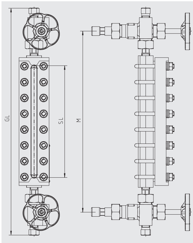
Ventilanordnung
