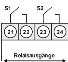
Klemme 2
