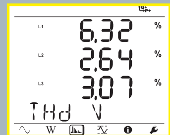
Klirrfaktor THD
