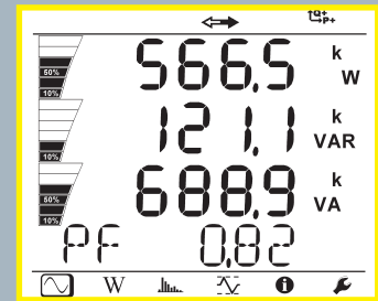
Leistung/P.F
