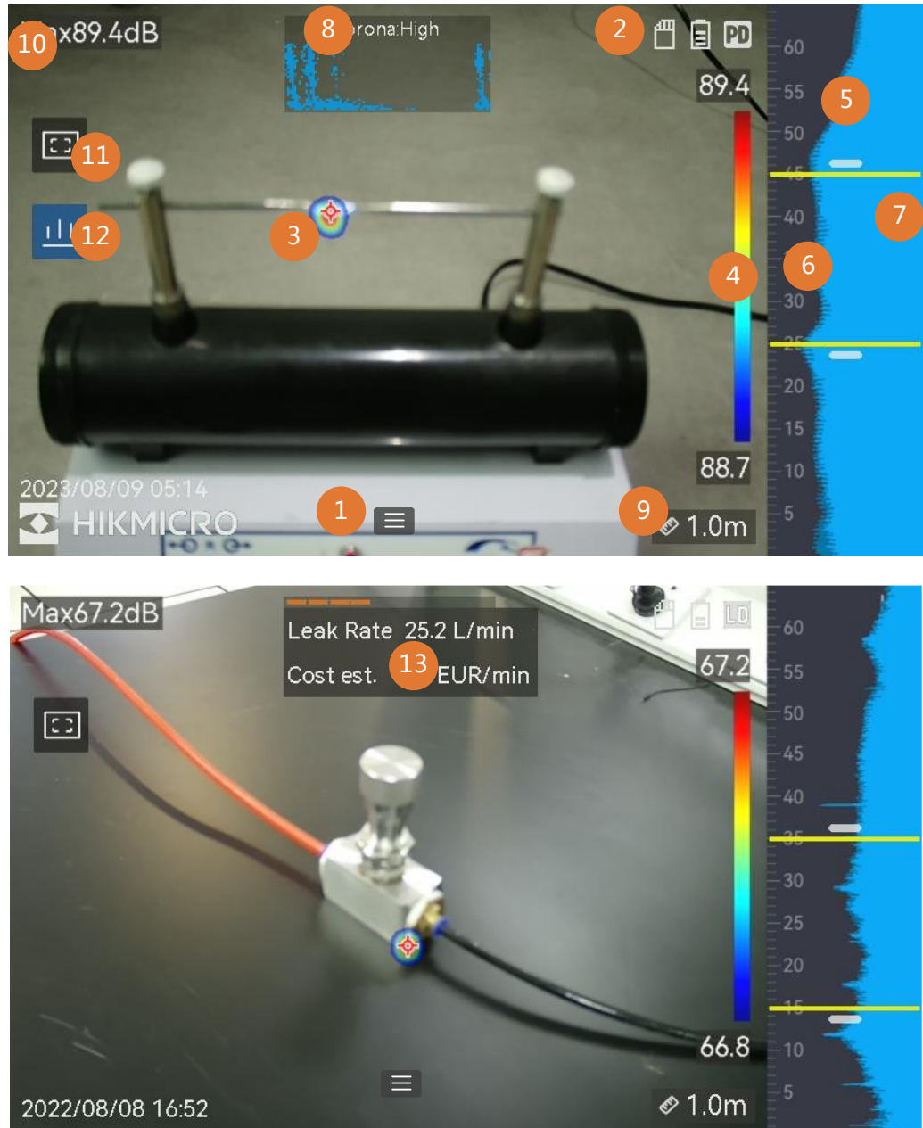
Abbildung 2-8 Live-Ansicht-Oberfläche
