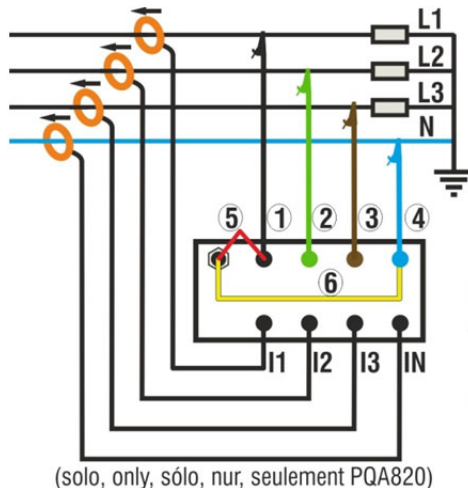
Abb. 4: Verbindung des Geräts in einem dreiphasigen System mit Neutraleiter
