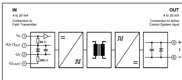
Prinzipschaltbild
