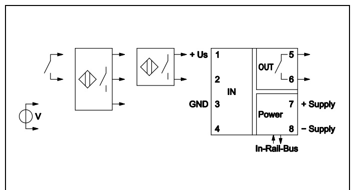
Prinzipschaltbild
