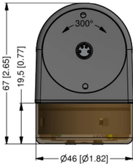
mit Stecker / Buchse M8x1
