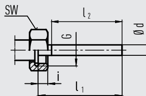
Bauform 3, Überwurfmutter
