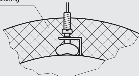
Winkeleisenhalterung Isolierung
