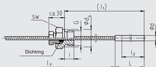
Bauform 6.3, Klemmverschraubung verschiebbar auf dem Spiralschutzschlauch (Klemmverschraubung nicht dichtklemmend)
