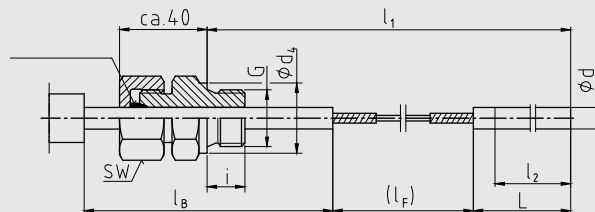
Bauform 7, Klemmverschraubung am Gehäuse
