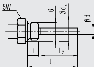
Standardbauform (Gewindeanschluss, fest)
