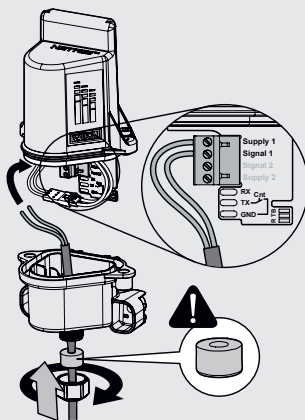
Conexión de una sola conexión analógica
