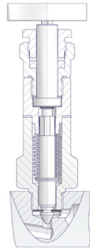
Ventiloberteil mit Faltenbalgdichtung
