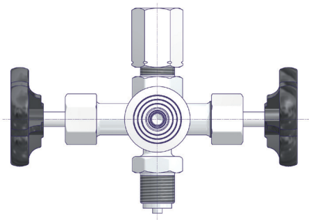
Ventil mit Prüfflansch \varnothing 40 \times 5
