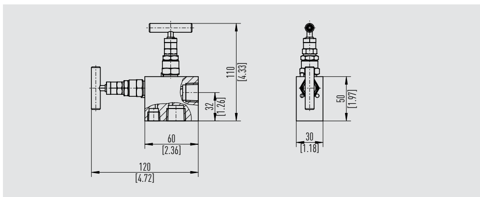
Typ IV2C1, flache Ausführung, gewinkelte Ventiloberteilstellung, integrierte Flanschmontage
