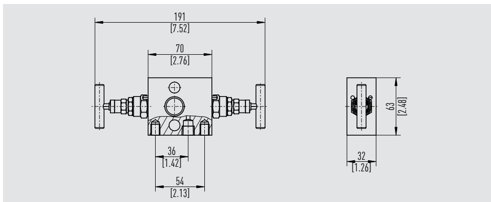
Typ IV2F7, flache Ausführung, L-förmige Ventiloberteilstellung, direkte Flanschmontage
