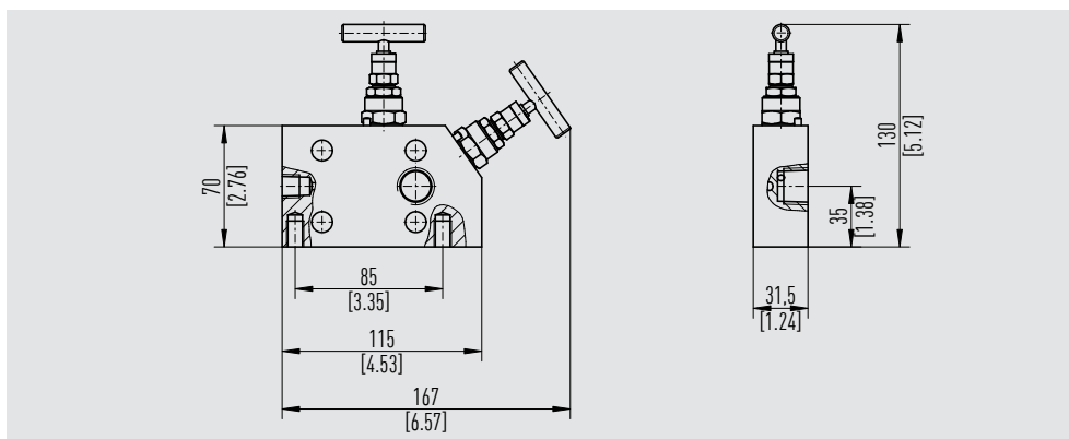
Typ IV2F2, flache Ausführung, In-Line-Ventiloberteilstellung, direkte Flanschmontage
